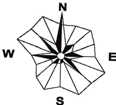
Дијаграм учесталости правца дувања ветра –ружса ветрова
